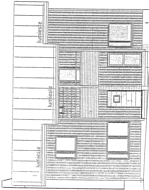
JULKISIVU 1
