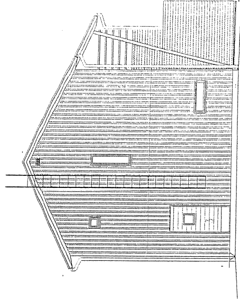
JULKISIVU 4
