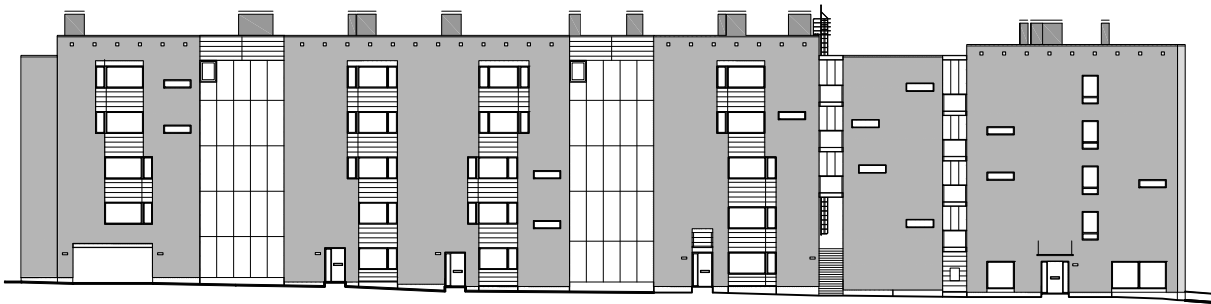
JULKISIVU POHJOISEEN
