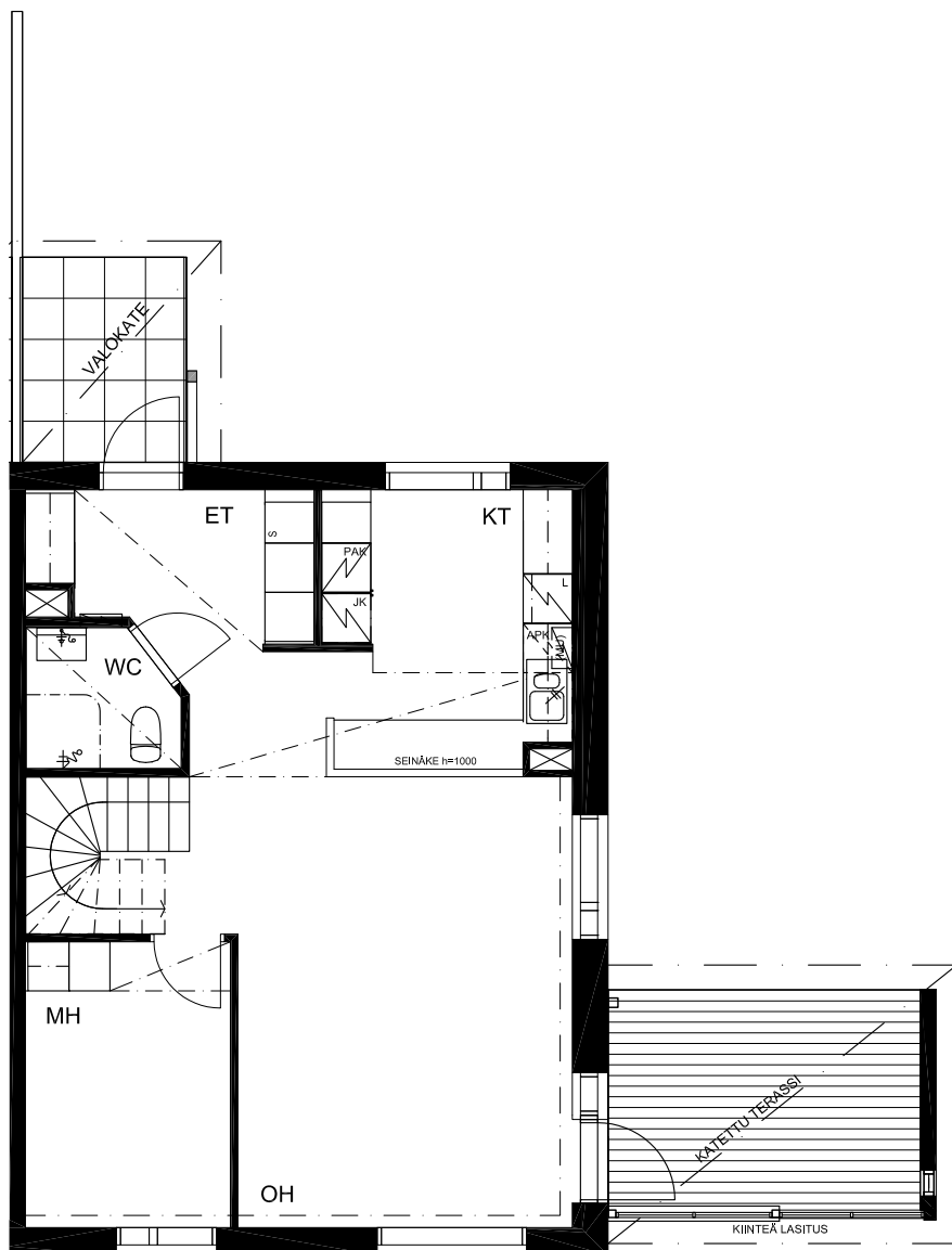
1. KERROS
