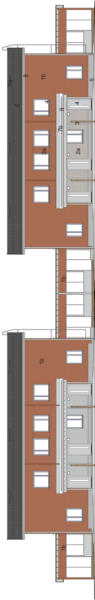
JULKISIVU ITÄÄN
