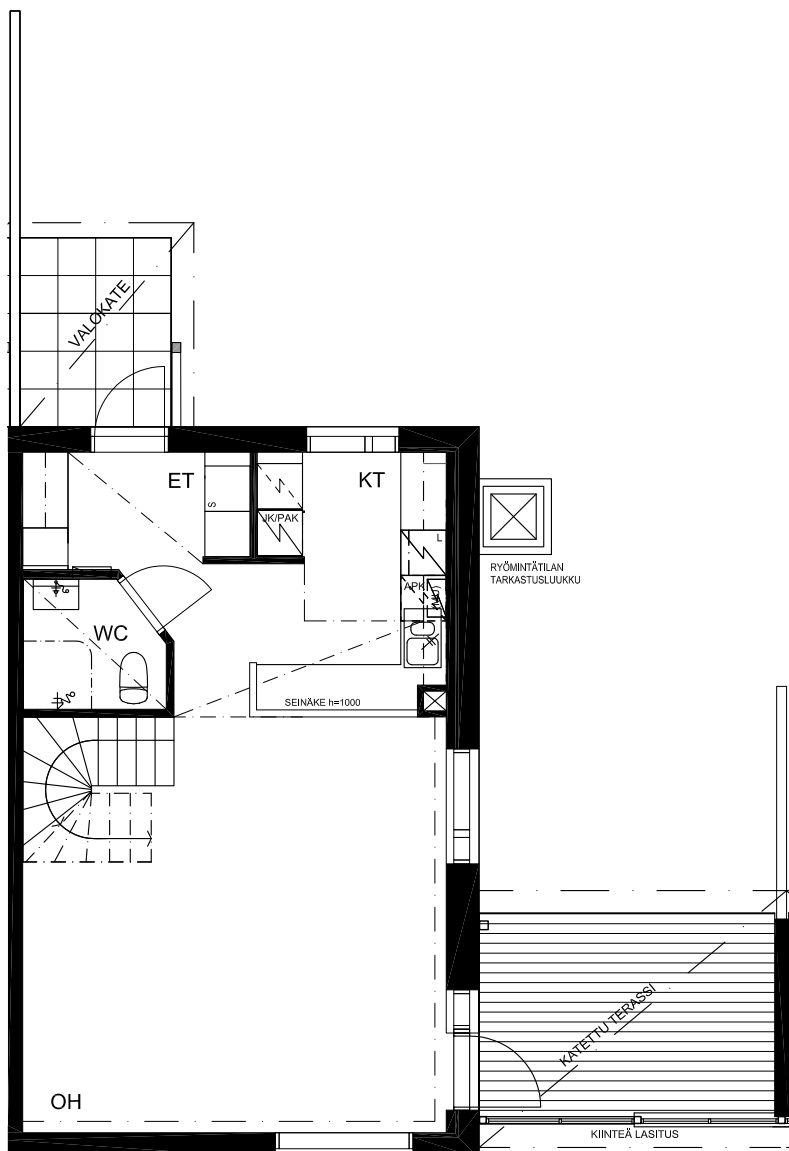
1. KERROS
