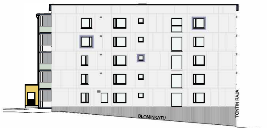
JULKISIVU ETELÄÄN
