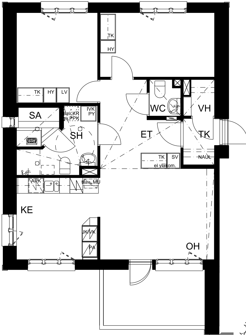
ASUNTO D28
