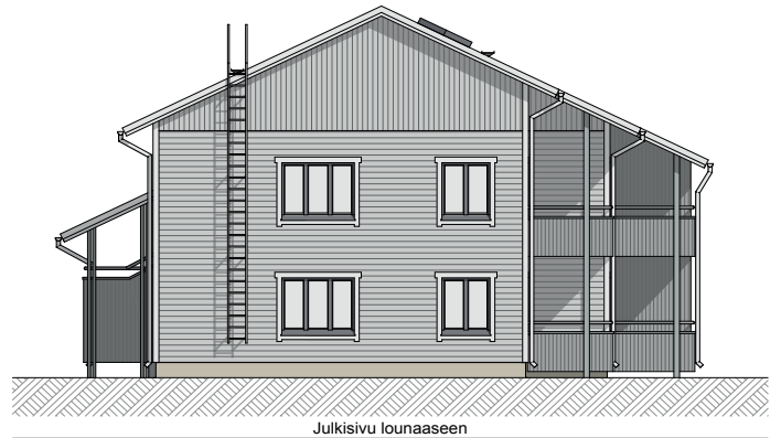
Julkisivu lounaaseen
