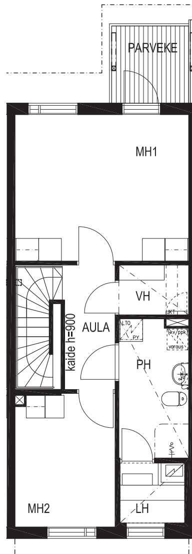
2. KERROS
