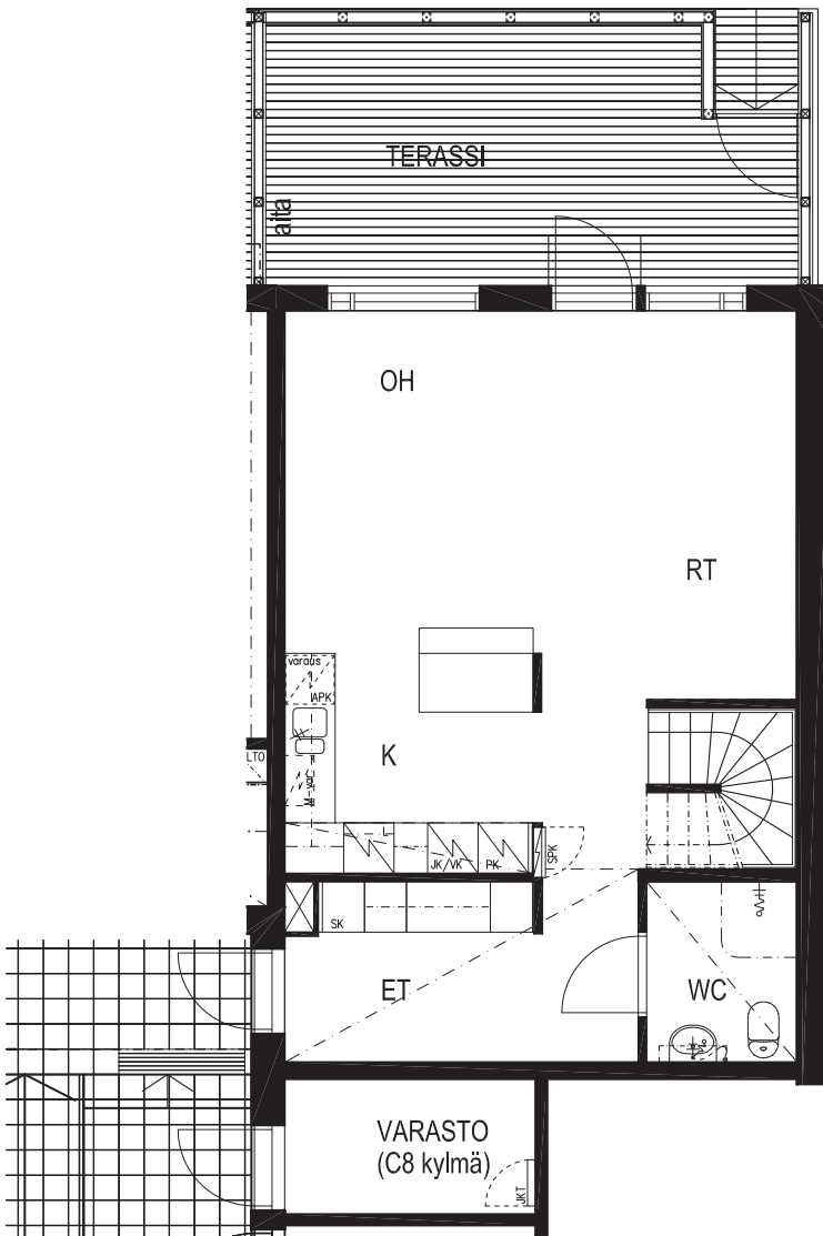
1. KERROS
