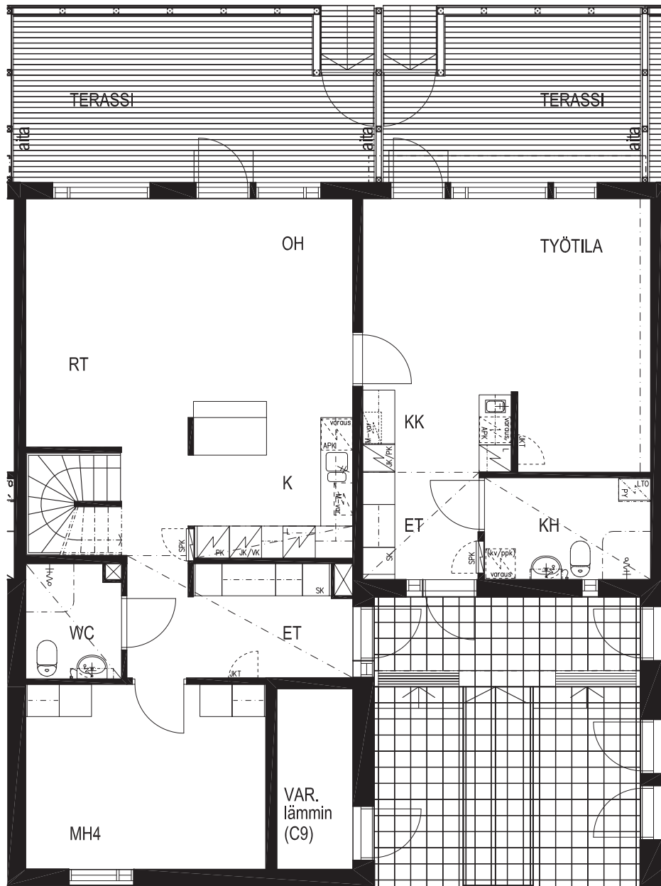
1. KERROS
