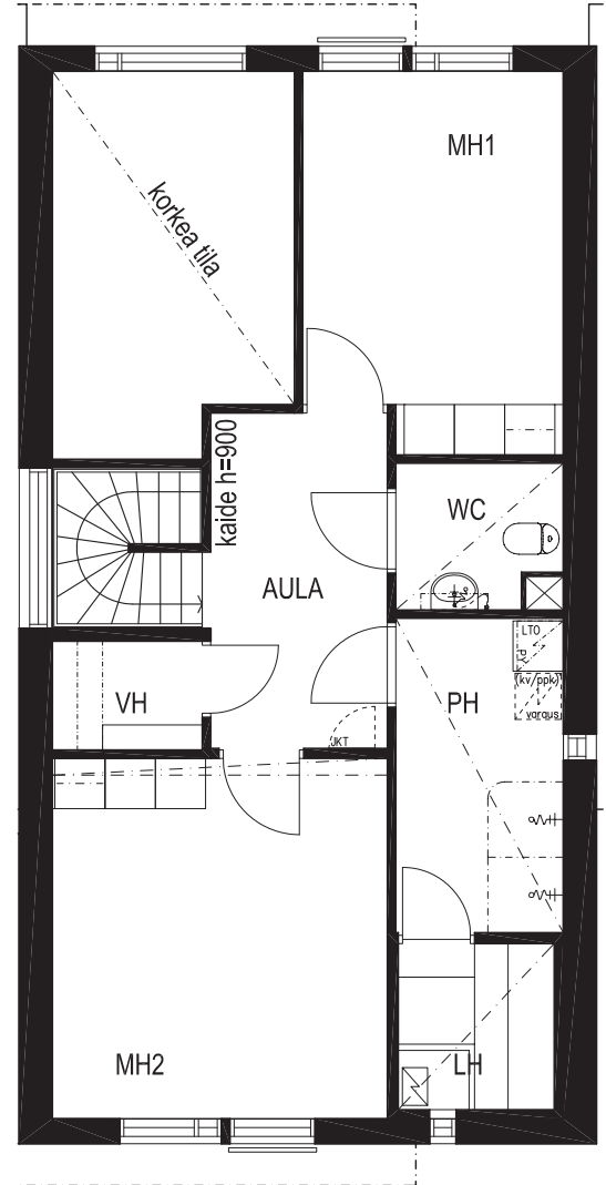
2. KERROS
