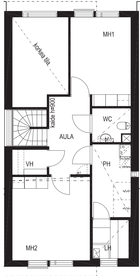
2. KERROS
