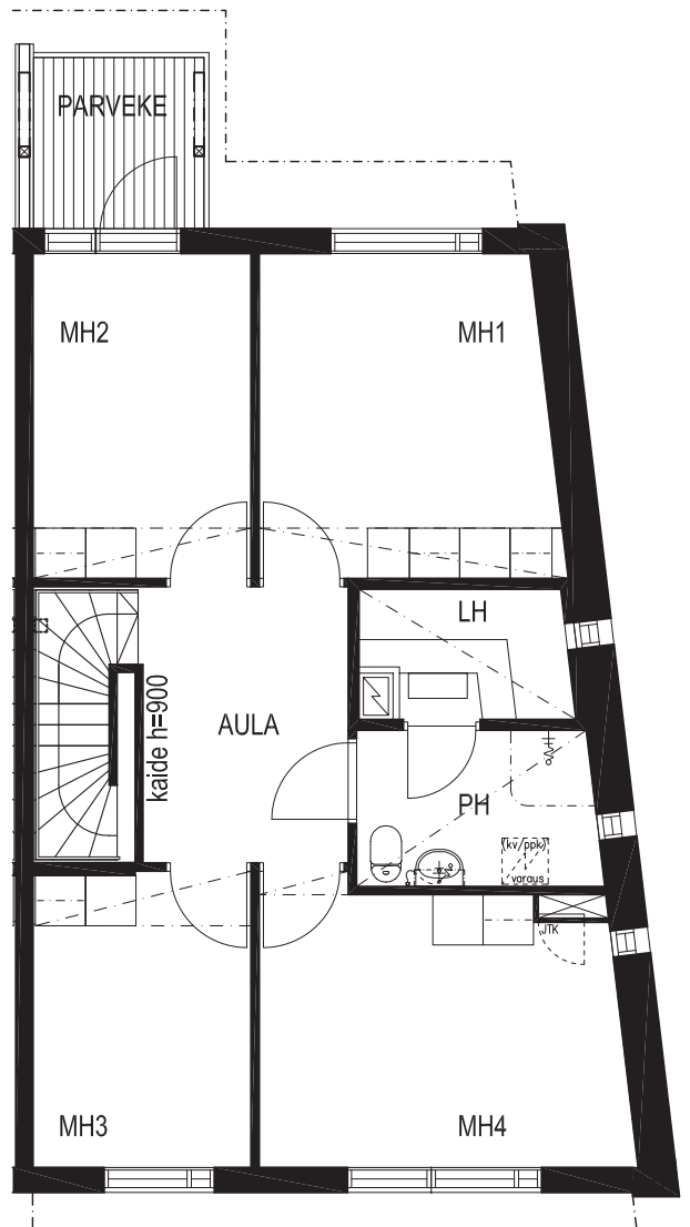
2. KERROS
