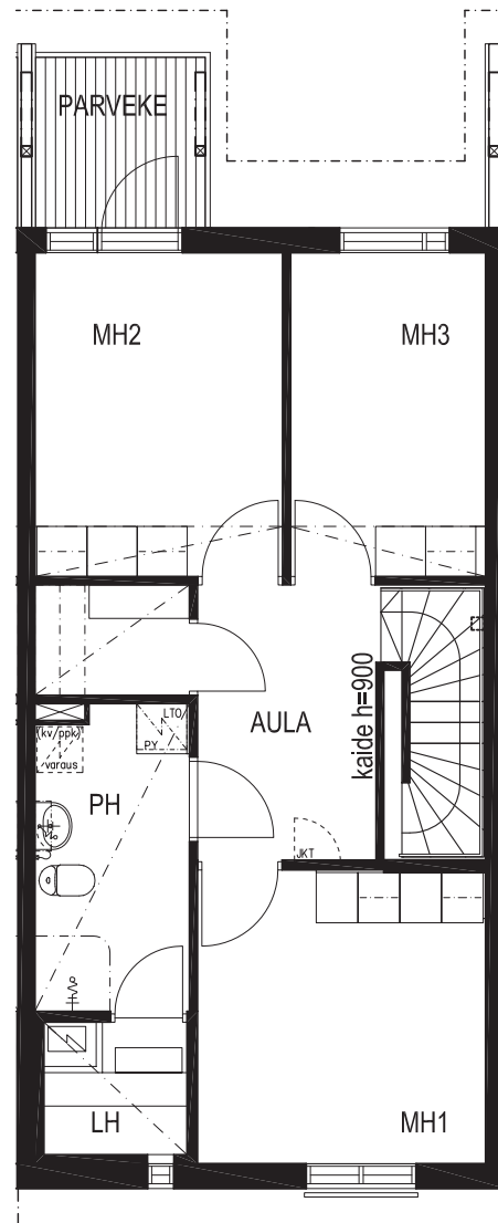
2. KERROS
