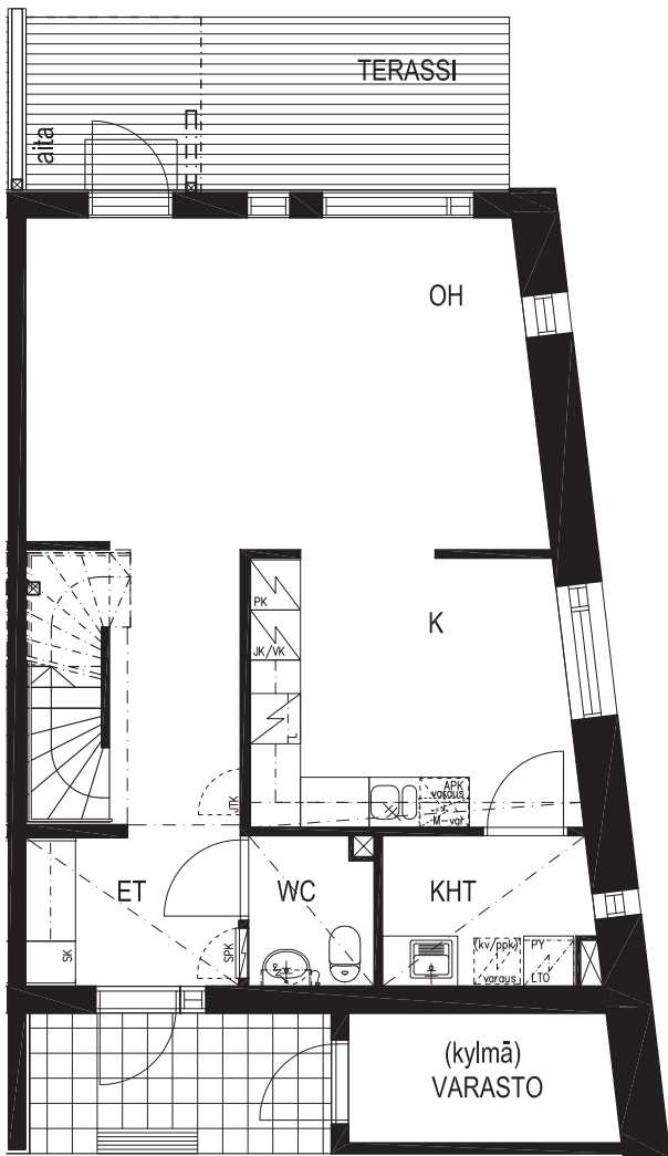
1. KERROS
