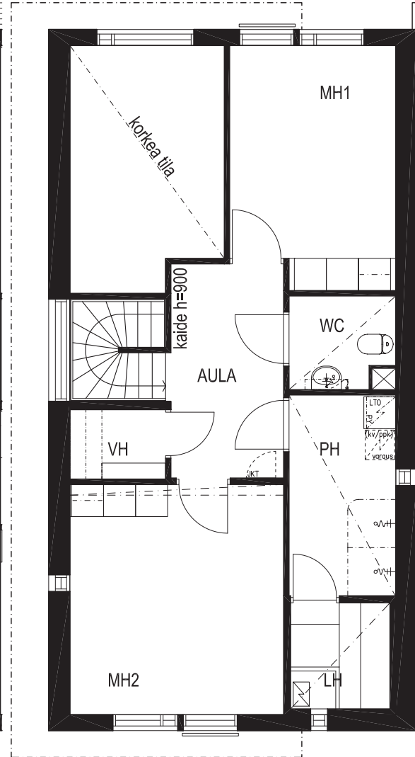
2. KERROS
