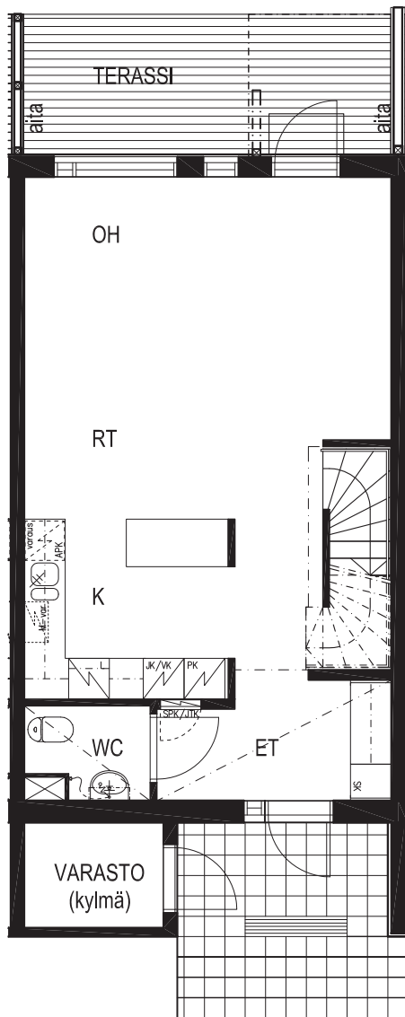
1. KERROS
