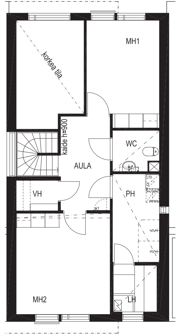
2. KERROS
