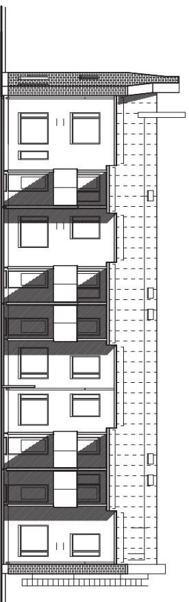
JULKISIVU ETELÄÄN
