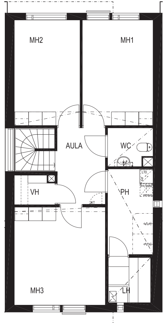
2. KERROS
