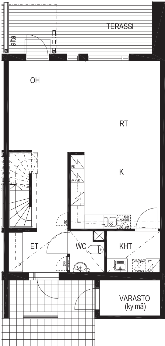
1. KERROS
