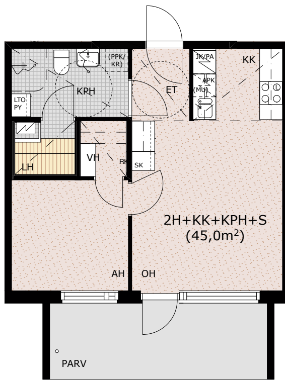
POHJAPIIRUSTUS
