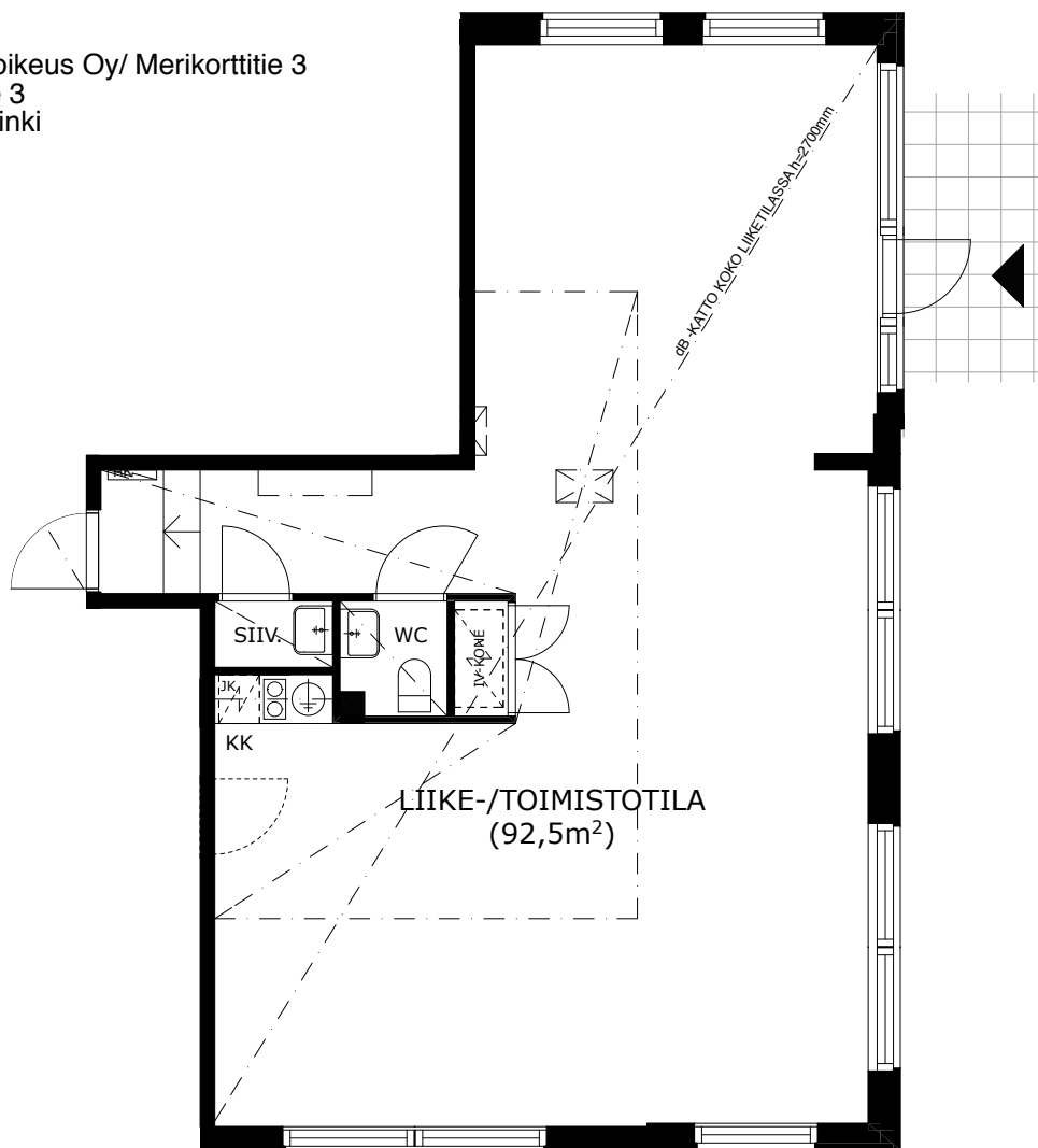
POHJAPIIRUSTUS
