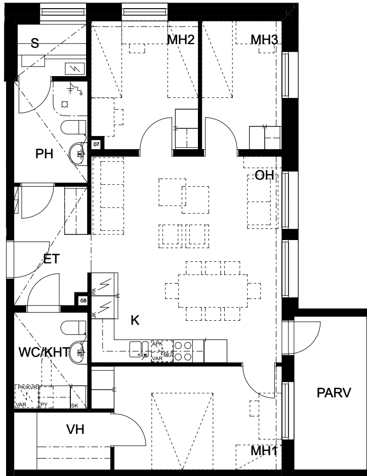
POHJAPIIRROS
