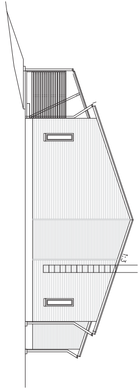
JULKISIVU ETELÄÄN
