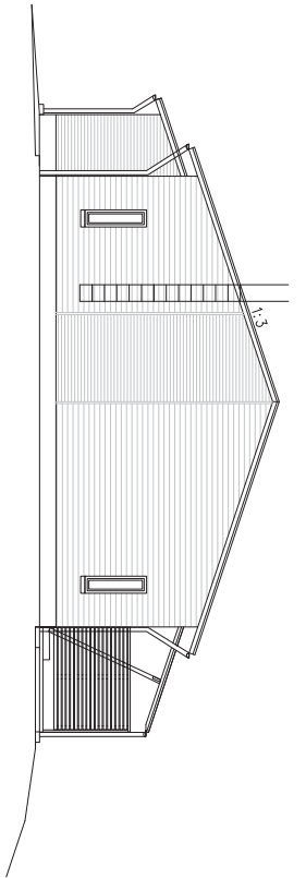
JULKISIVU POHJOISEEN
