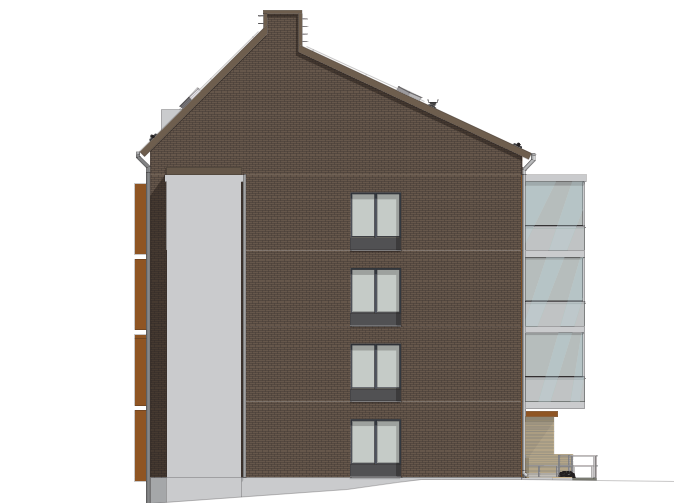
Julkisivu / länsi
