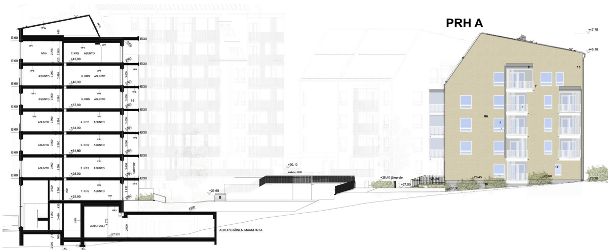
PIHAJULKISIVU LOUNAASEEN
