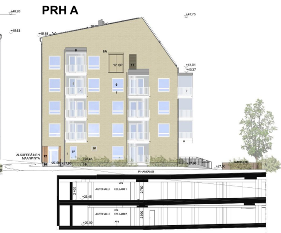
PIHAJULKISIVU KOILLISEEN
