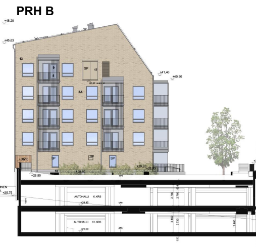
PIHAJULKISIVU POHJOISEEN
