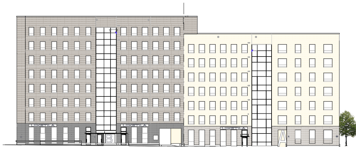
JULKISIVU ITÄÄN KONALANTIELLE B
