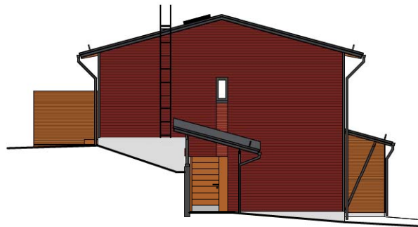
julkisivu länteen
