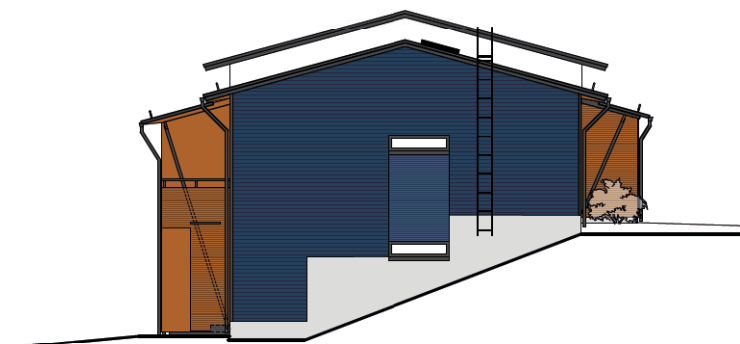
julkisivu itään
