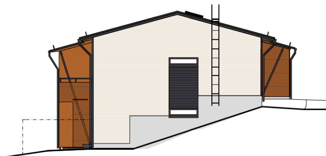
julkisivu itään
