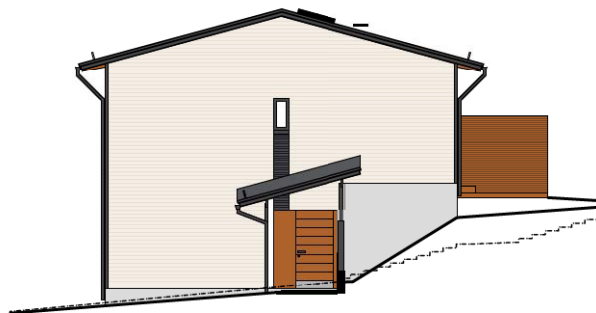
julkisivu itään
