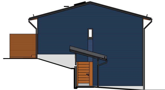
julkisivu länteen
