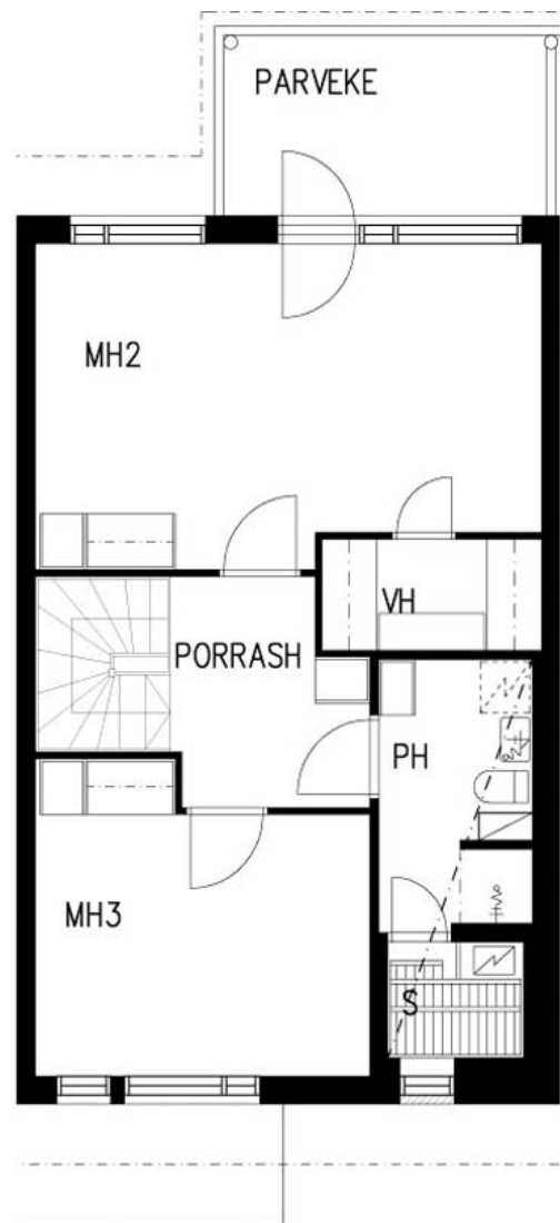
2. KERROS
