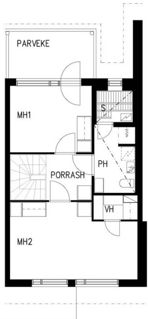
2. KERROS
