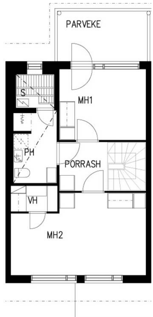
2. KERROS
