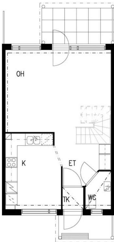
1. KERROS
