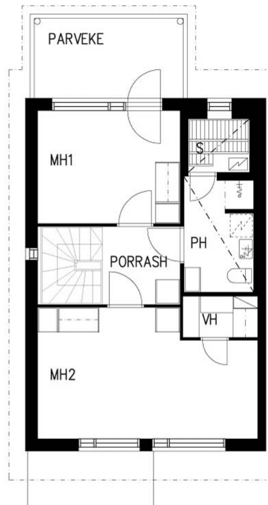
2. KERROS
