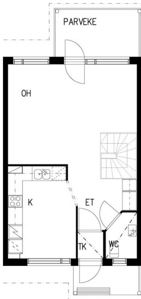
1. KERROS
