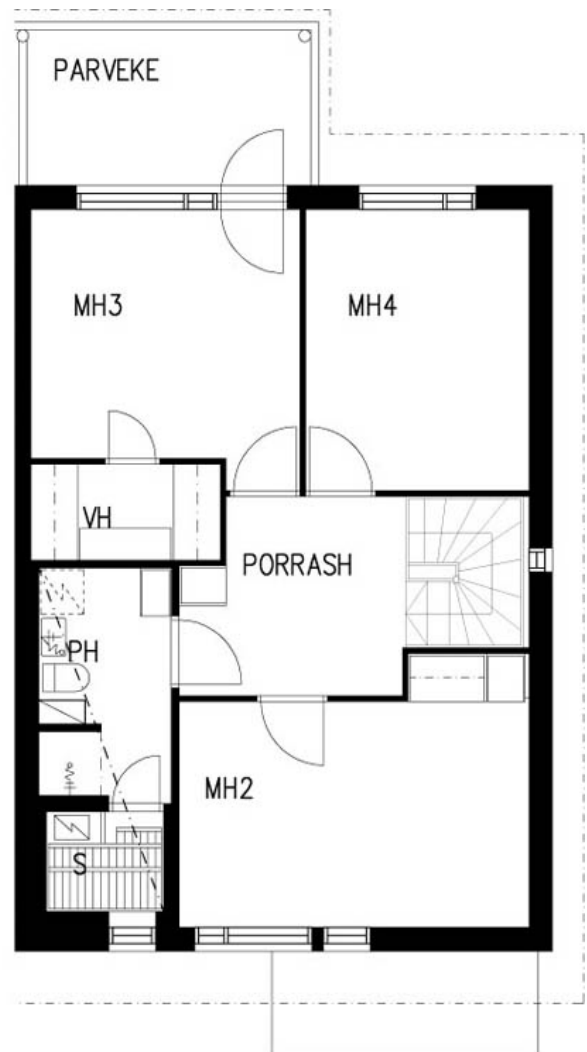
2. KERROS
