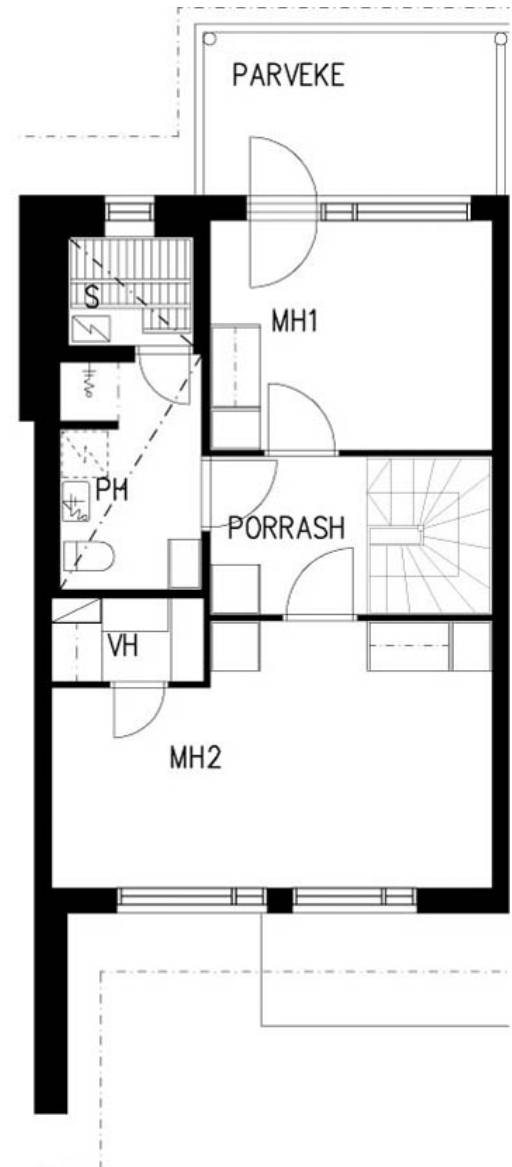
2. KERROS
