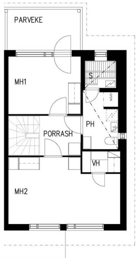
2. KERROS
