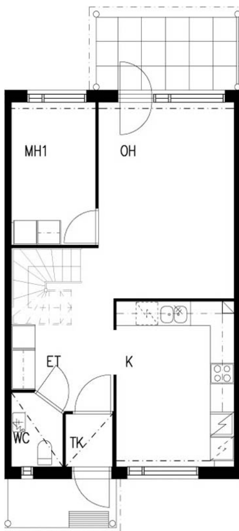
1. KERROS
