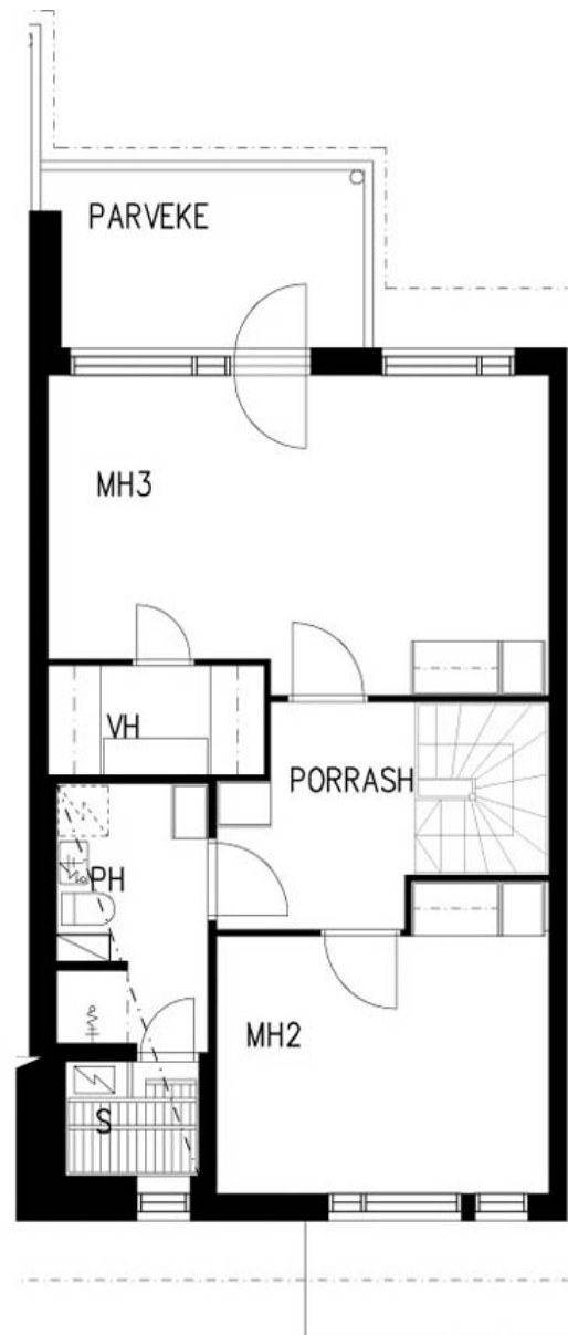
2. KERROS
