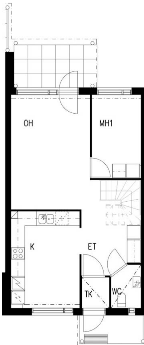
1. KERROS
