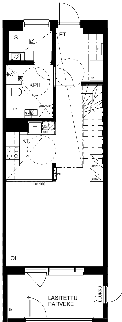
B36 alakerta 1 : 100
