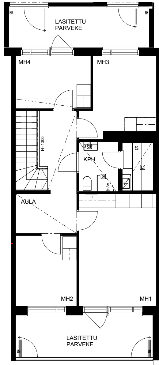
B30 yläkerta 1 : 100
